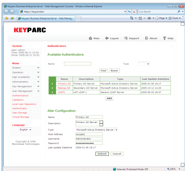
Keyparc Business 企业版服务器管理控制台
